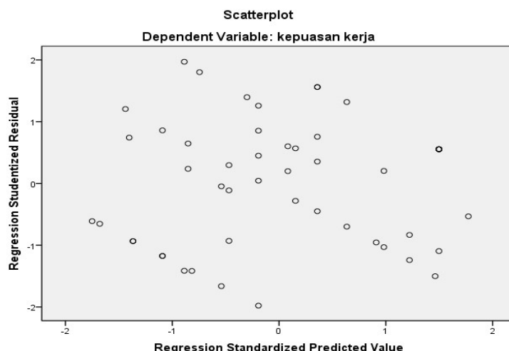
Gambar 1. Uji Heteroskedastisitas
